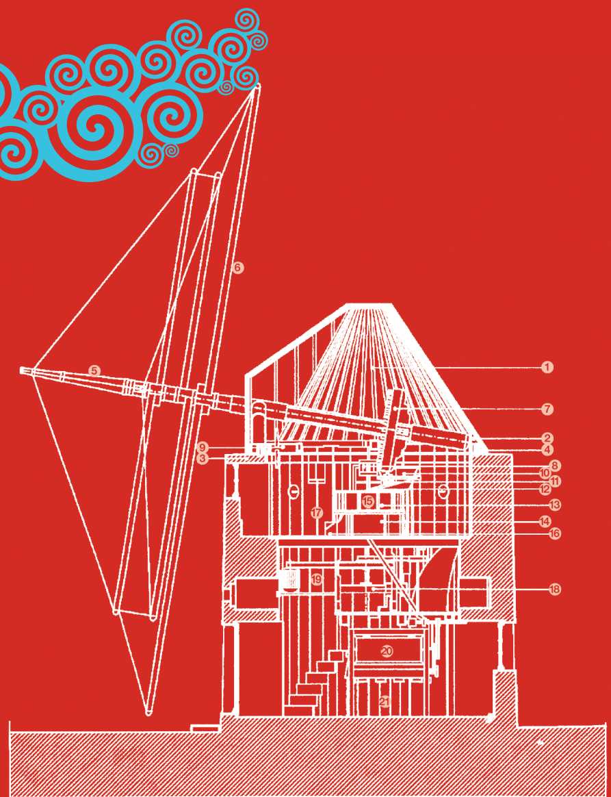
CORTE ESQUEMÁTICO DO MOINHO DA FORÇA
